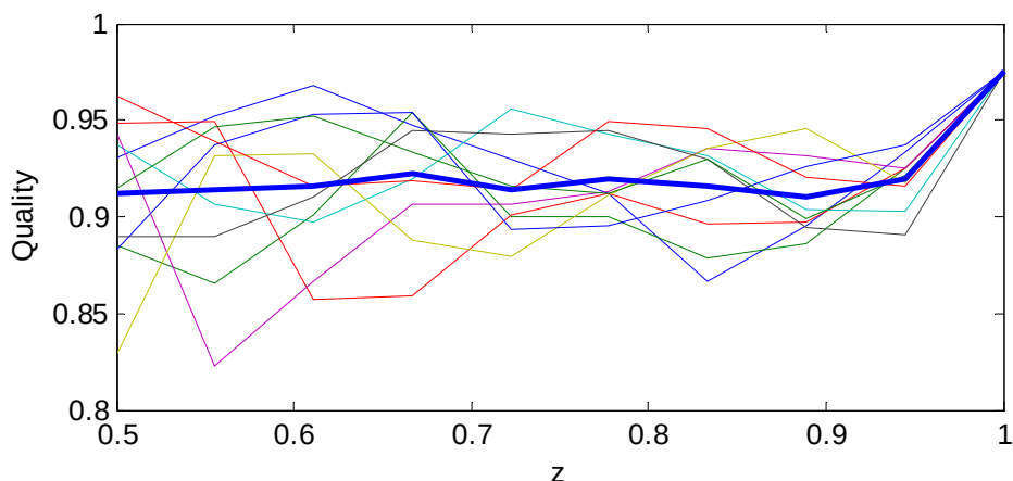
Рис. 4.2.2. Качество классификации в первой серии экспериментов.
