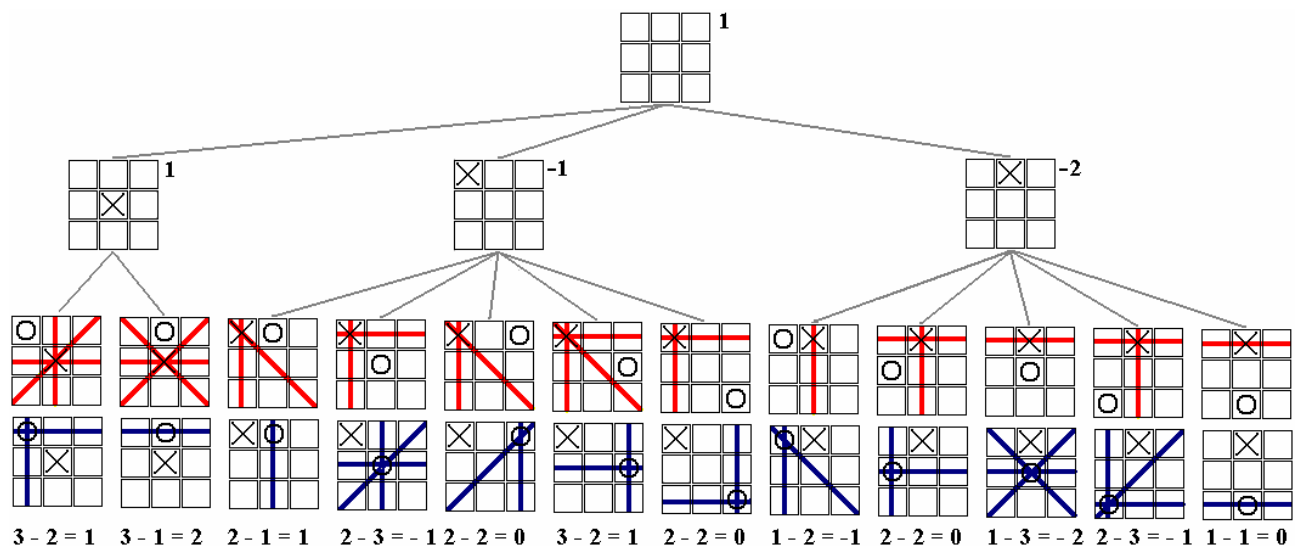
Рис. 1.2.1. Применение простой функции оценки в «крестиках-ноликах».
