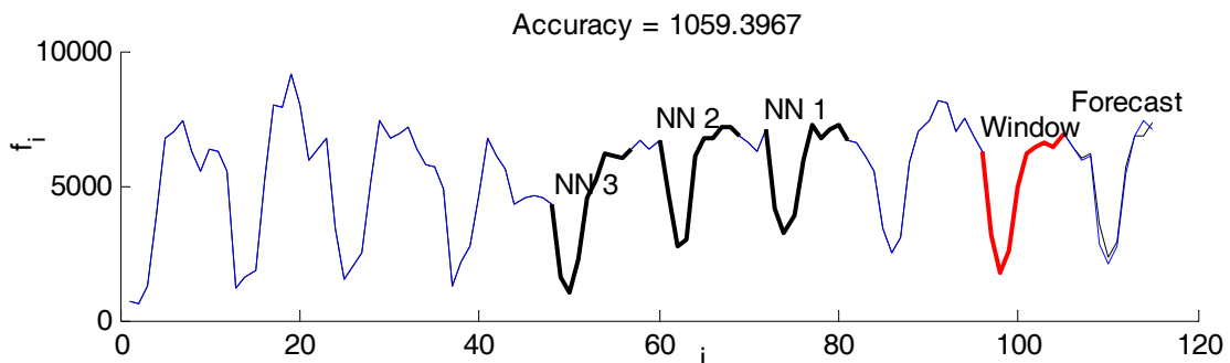
Рис. 12.4.4. Прогнозирование реального ряда с тремя соседями.
