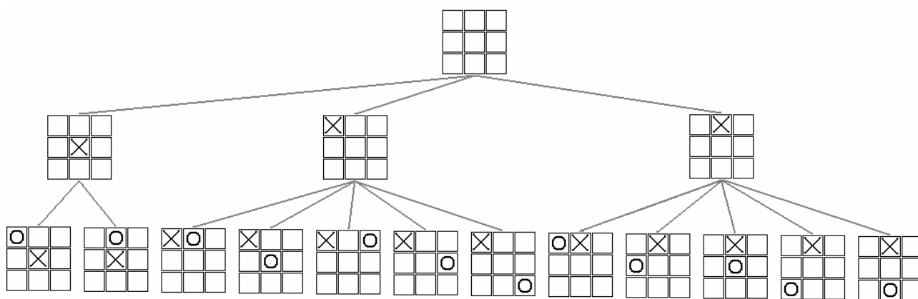
Рис. 1.1.4. Первые уровни дерева игры крестики-нолики 1 .
