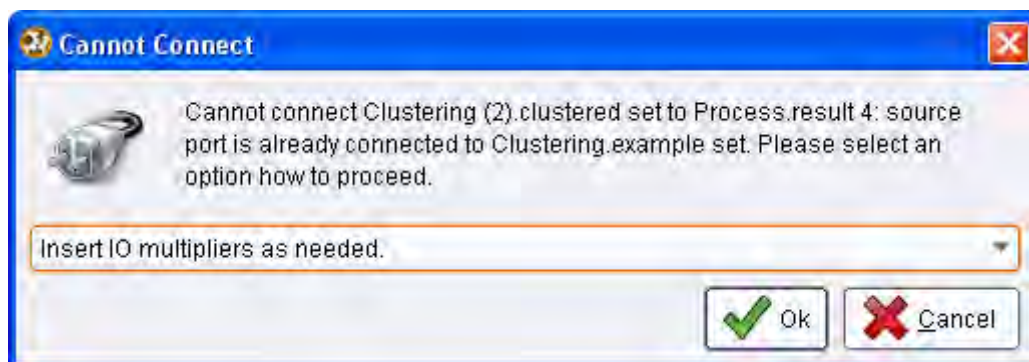
Рис. 14.4.4. Разветвление связей.
