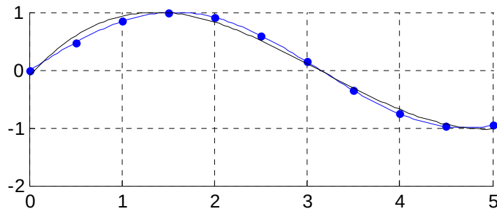
Рис. 7.2.1. Полиномиальная регрессия.
