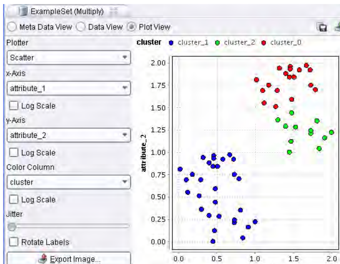
Рис. 14.4.6. Визуализация кластеризации.
