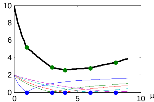
Рис 3.3.3. График функции (3.3.5).
