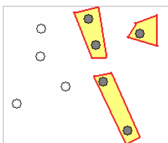
Рис. 6.4.2. Эффект переобучения.
