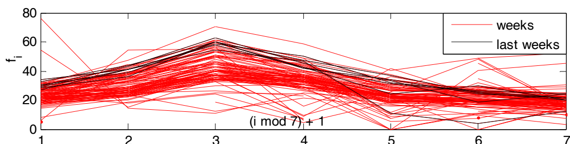
Рис. 12.4.11. Ряд рис. 12.4.10, записанный «по неделям».
