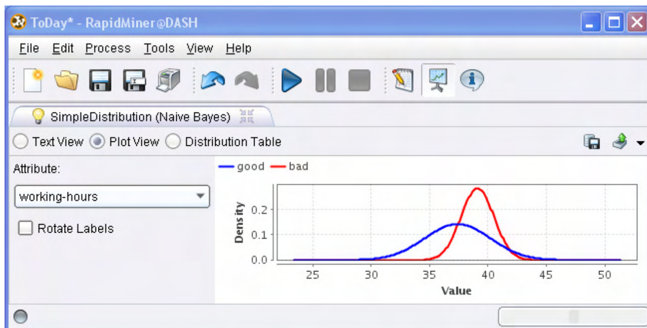
Рис. 14.3.3. Построение байесовского классификатора.
