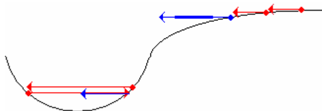
Рис. 6.2.3. Идея эвристики delta-bar-delta.
