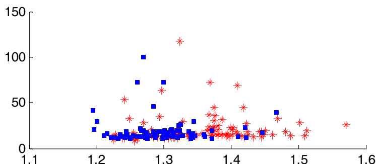
Рис. 12.1.5. Результат ShowFs(mean(abs(diff(X'))), mean(abs(X')), Y) .
