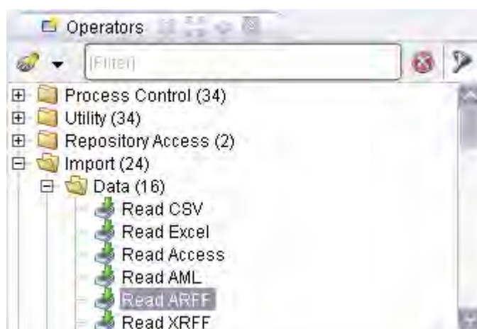
Рис. 14.2.1. Панель Operators.
