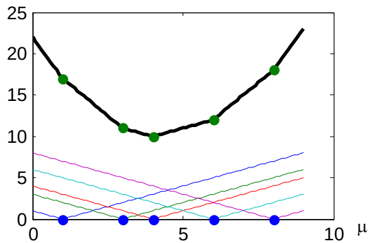
Рис 3.3.1. График функции (3.3.3).
