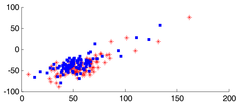
Рис. 12.1.3. Результат ShowFs(max(X'),min(X'),Y) .
