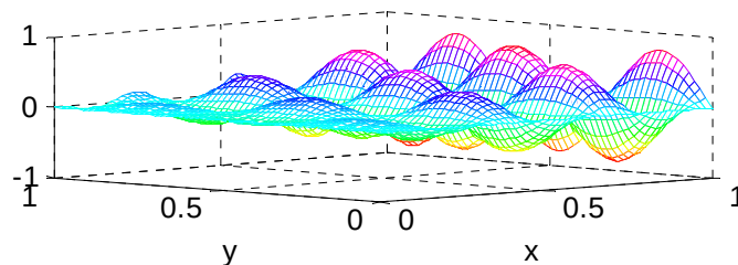
Рис 8.1.2. Функция \sin(x) \cdot \sin(20x) \cdot \sin(10y) .
